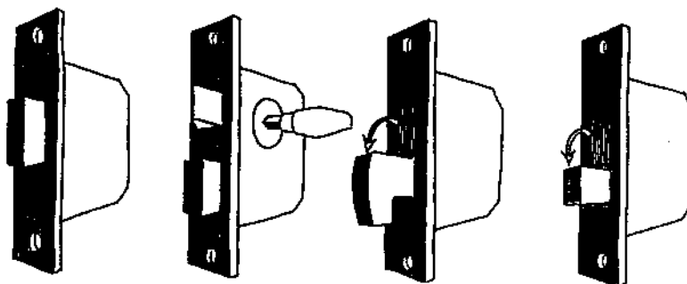
Reilelås
